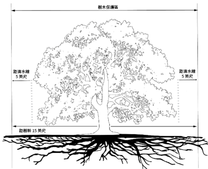
圖2：保護區（立面圖）
